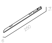
SPS Con Line 250 0330 PB DIM
